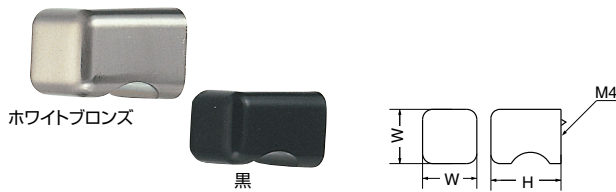
KZ-19 角キャノンツマミ (亜鉛合金/ISO4×28)
