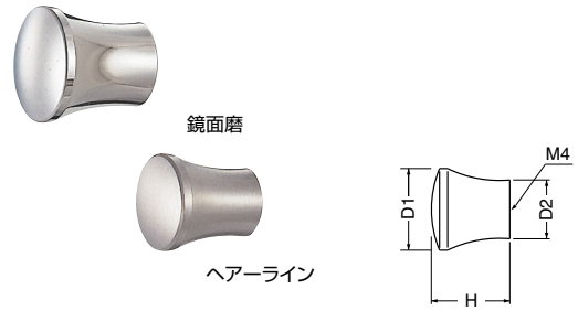
ST-80 ステンルーシートツマミ (ステンレス/4×28)
