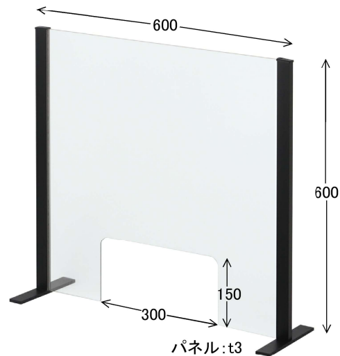
書類などのやり取りに便利な切り欠きタイプ
