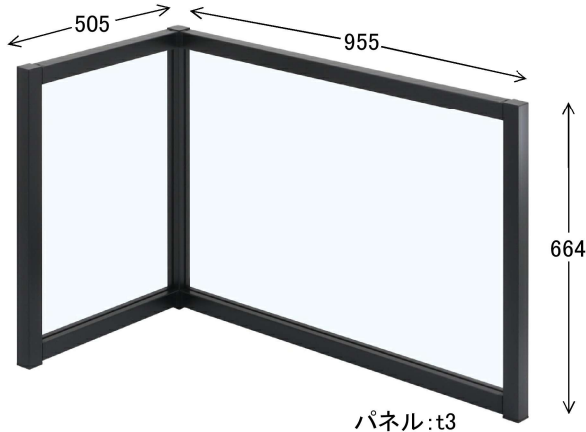
2方向からの飛沫防止に役立つL形タイプ
