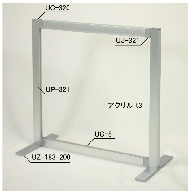
UC-320 エンドキャップ (ABS)
