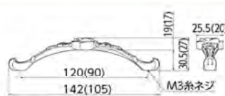
HB-350 プリンセスローズハンドル
